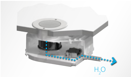
Un boîtier d'encastrement en technopolymère, muni de barres de renfort pour assurer le passage de véhicules et conçu pour favoriser l'écoulement de l'eau par un système WATER DRAIN, est proposé comme accessoire
